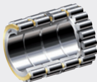
Roulements à plusieurs rangées de rouleaux cylindriques de NKE
