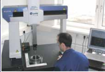
^ CNC koordináták mérőrendszere
